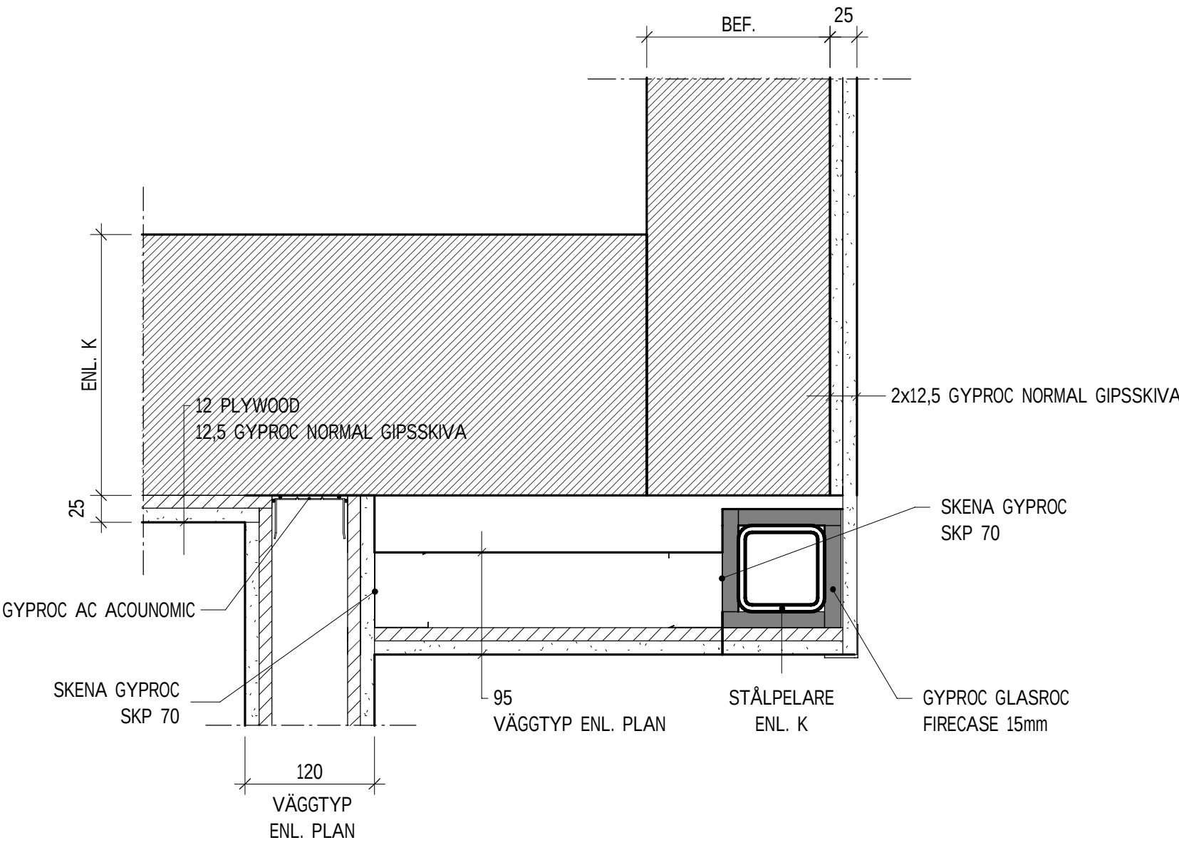
IK9 - STÅLPELARE VID BEFINTLIG VÄGG 1 : 5
