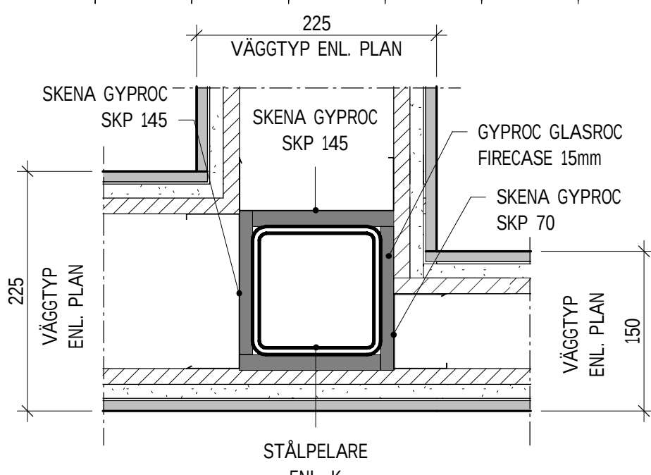
IK7 - STÅLPELARE I VÄGGKORSNING KÖK 1 : 5
