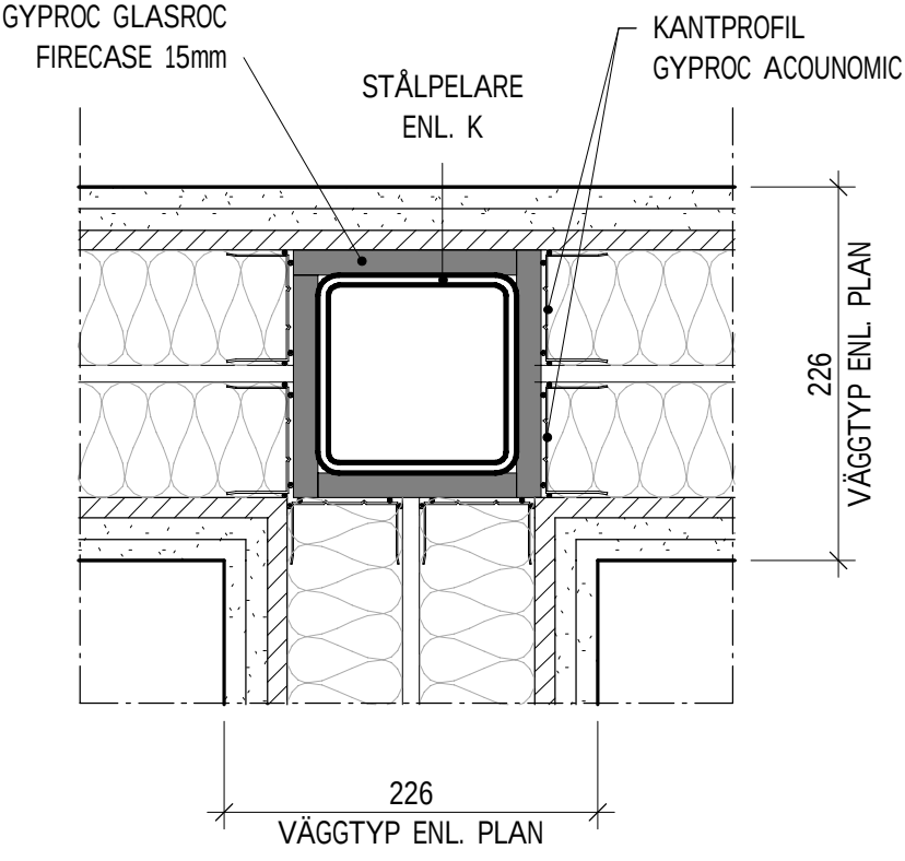
IK4 - STÅLPELARE I VÄGGKORSNING 1 : 5
