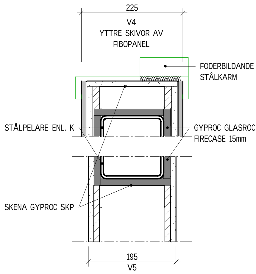
IK2 - STÅLPELARE I INNERVÄGG 1 : 5
