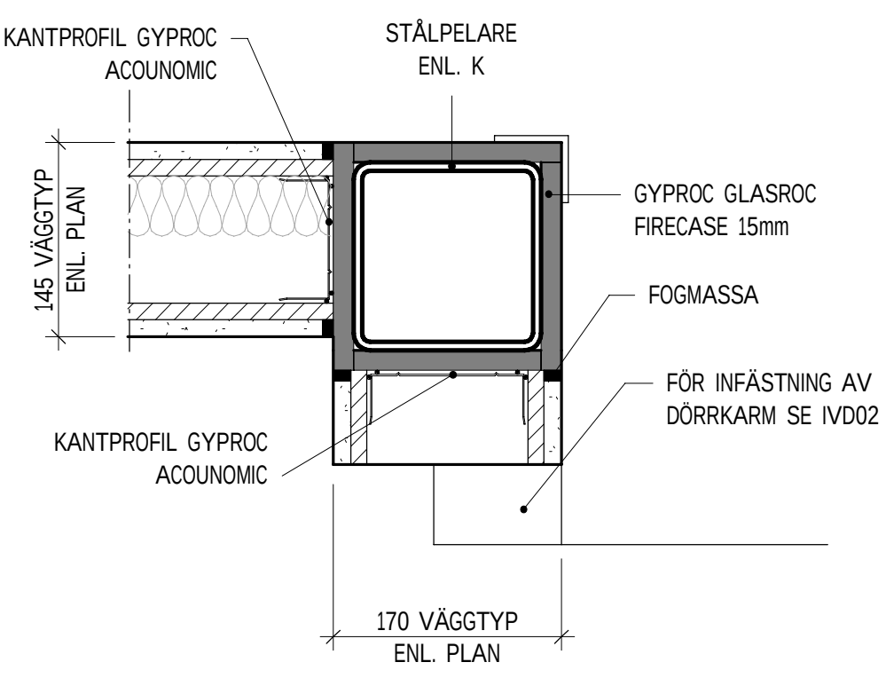
IK5 - STÅLPELARE I INNERVÄGGSHÖRN 1 : 5
